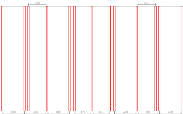
FASE 2: aggiunta di montanti in corrispondenza delle porte o moduli vetrati
