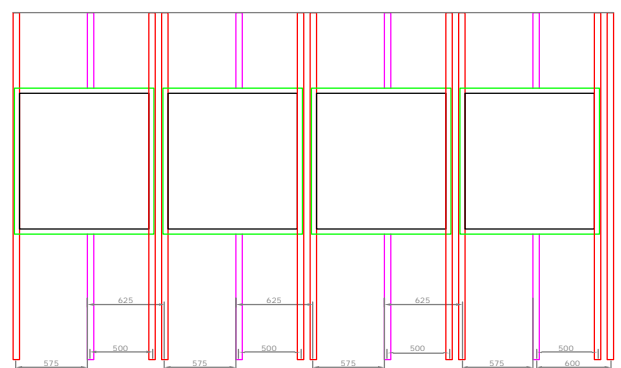
FASE 3: montaggio moduli e inserimento degli spezzoni dei montanti con passo 60 cm. in corrispondenza dei moduli vetrati
