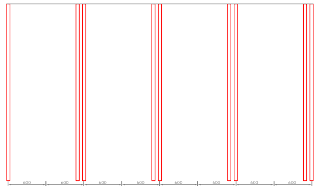
FASE 2: spostamento di montanti in corrispondenza delle porte o moduli vetrati
