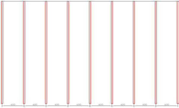
FASE 1: montaggio montanti ogni 60 cm.
