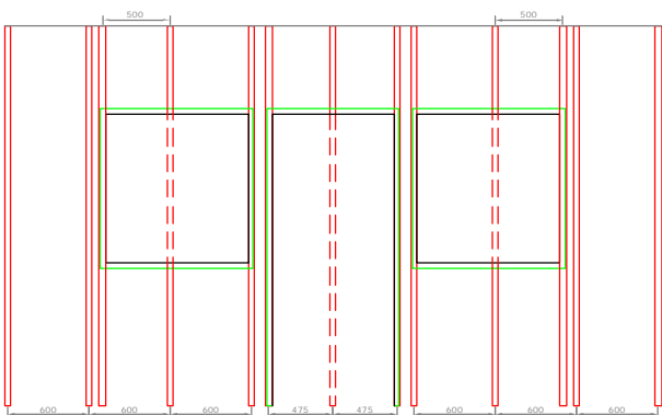
FASE 3: montaggio porte e moduli e taglio dei montanti in corrispondenza degli stessi
